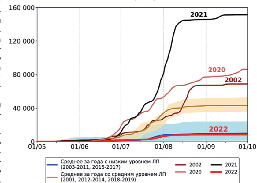
Кол-во термоточек в Якутии (нарастающий итог с начала года) MODIS (Terra)
