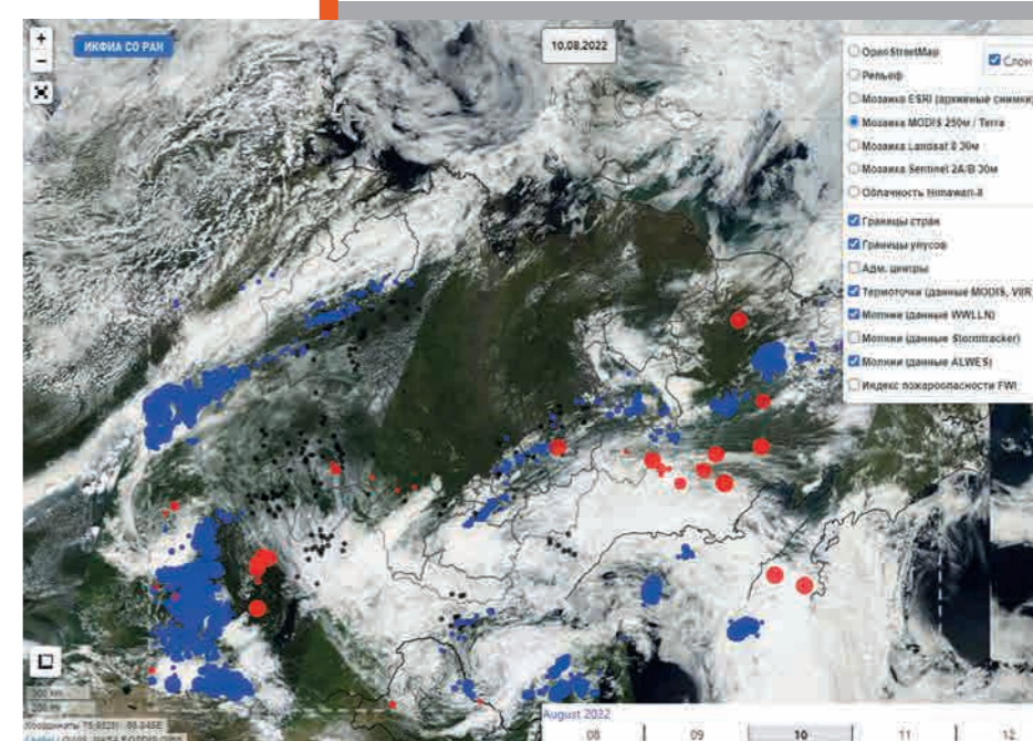
Рис. 1. Обстановка на 10 августа 2022 г. Интерфейс Интернет-ресурса информационной поддержки лесопожарного мониторинга с отображением тематических слоев – облачность по данным прибора MODIS (250 м), карта термоточек (данные MODIS, VIIRS), карта молниевых разрядов (данные грозопеленгационных сетей ИКФИА и WWLN)
